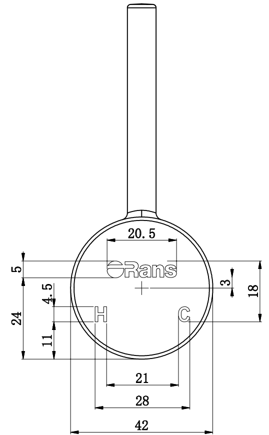
把手 比例 1.000
